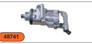
Гайковерт пневматический ударный, 1"DR, 5000 об/мин, 2430 Nm. JAI 1138
