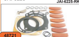
Ремонтный комплект для пневматического гайковерта JAI-6225 JAI-6225-RK
